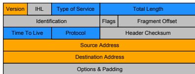
IPv4-header
